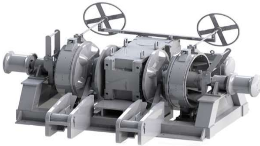
Gambar 1. Mesin windlass dengan penggerak tenaga listrik
