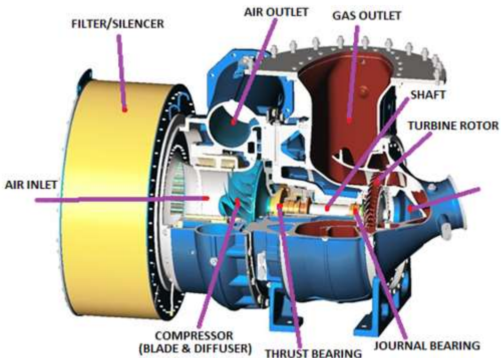
Gambar 1 Penampang dan Bagian-Bagian Turbocharger
