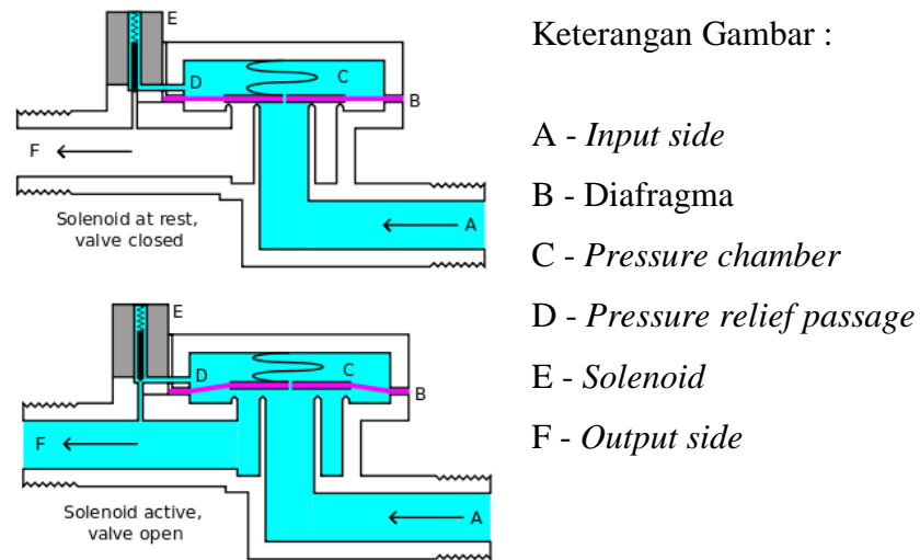
Gambar 5. Bagian-bagian Dari Solenoid Valve (Sumber : www.solenoidvalve.com . [04-03-2019])
