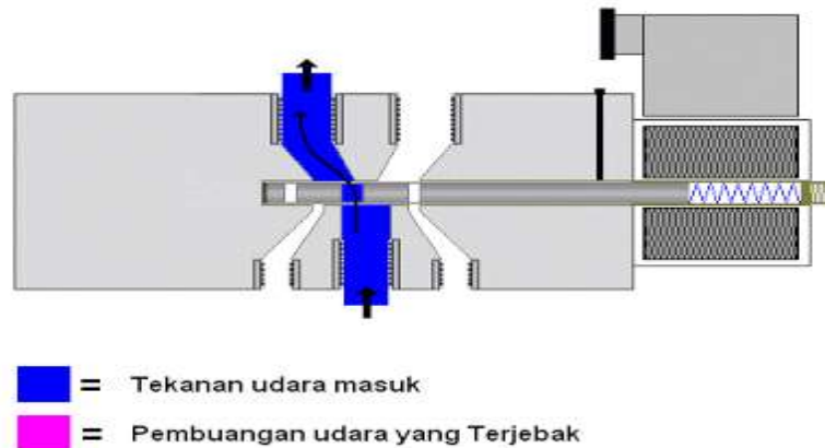
Gambar 8. Skema Langkah Kerja Solenoid Valve
