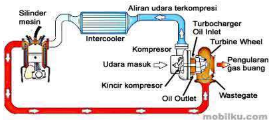
Gambar 2.3 Aliran Udara Bilas Pada Turbo
