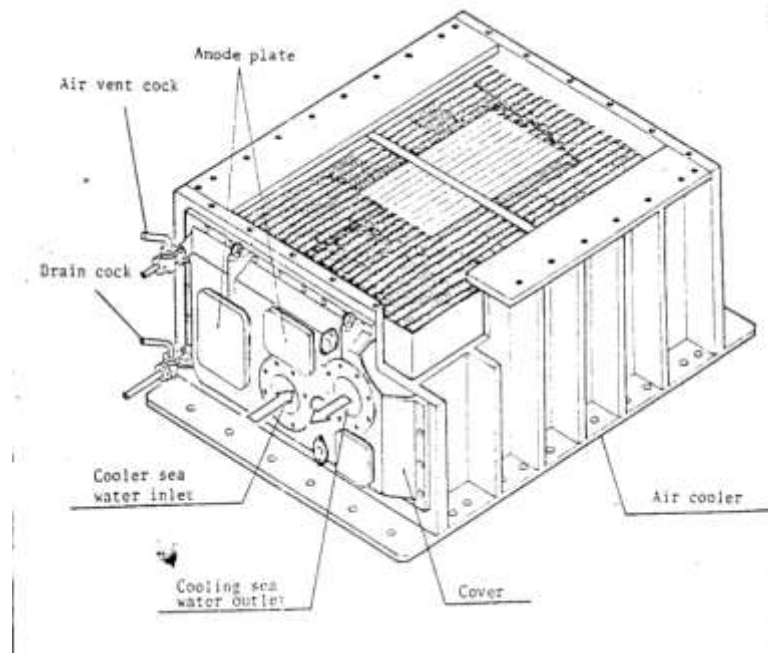
Gambar 2.1 Bagian Bagian Intercooler Mesin Induk
