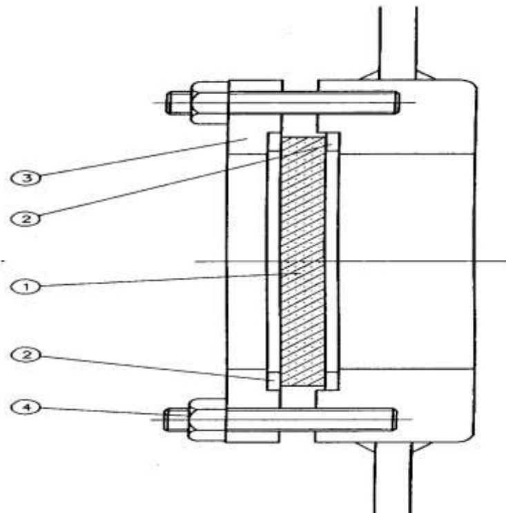
Gambar 12 Gambar gelas duga
