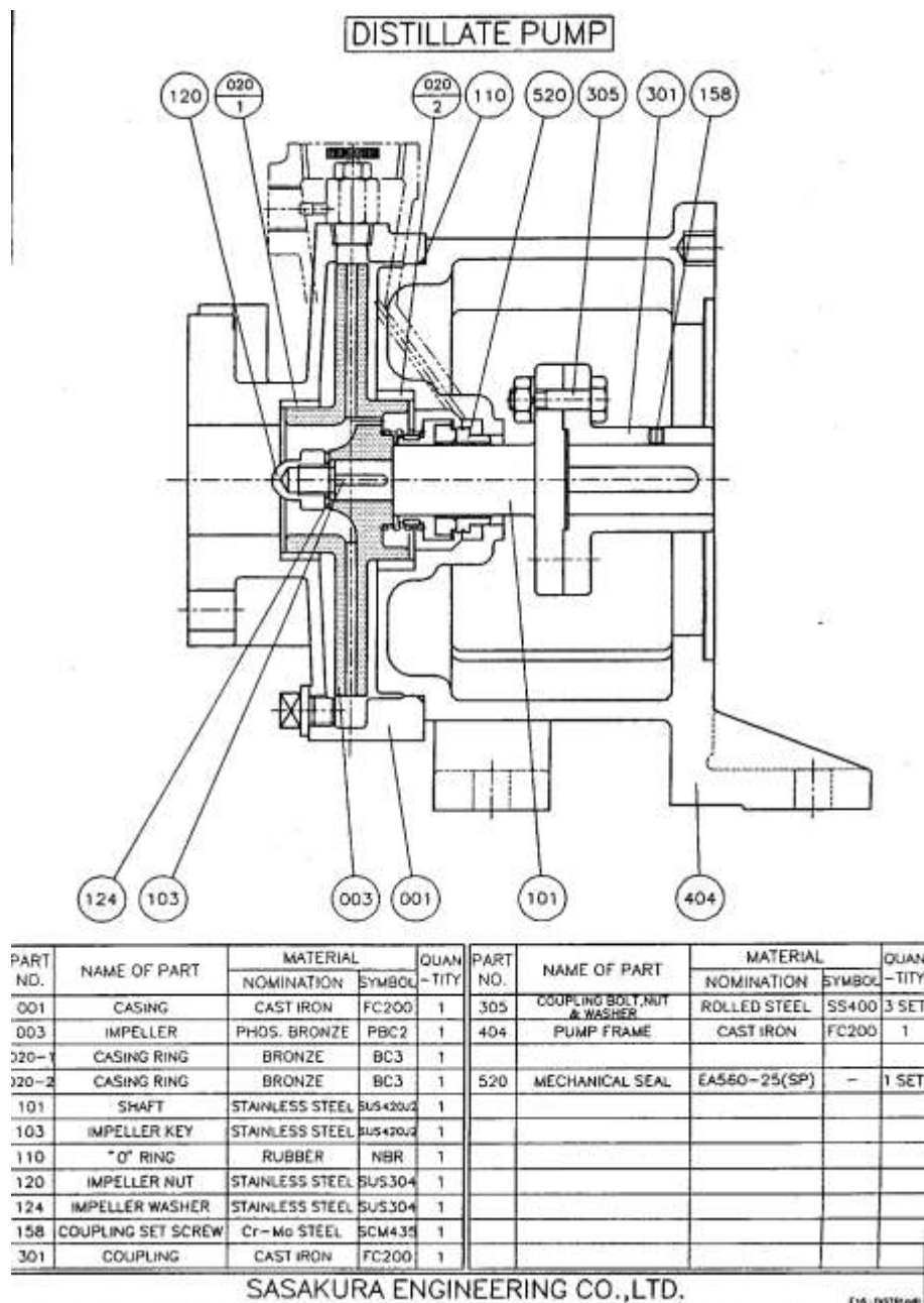
Gambar 7 Bagian bagian pompa distillate
