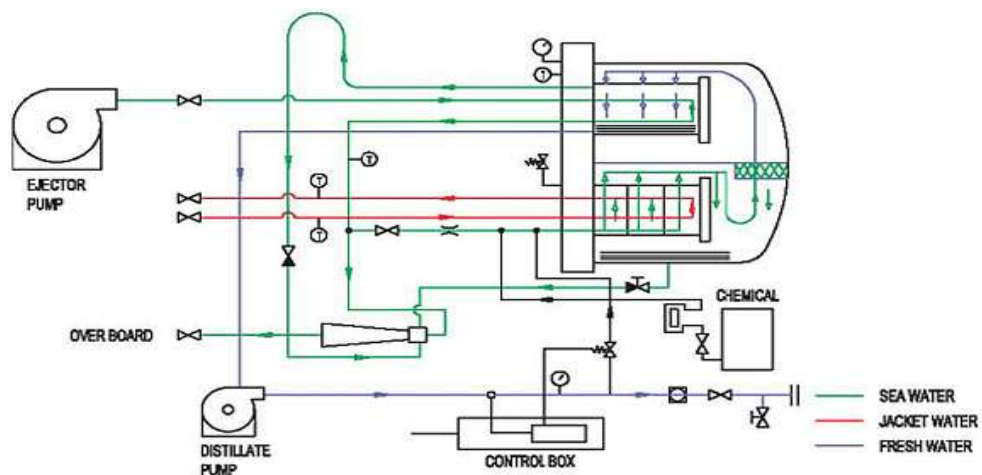
Gambar 3 proses aliran air laut dan air tawar dalam proses Fresh Water Generator
