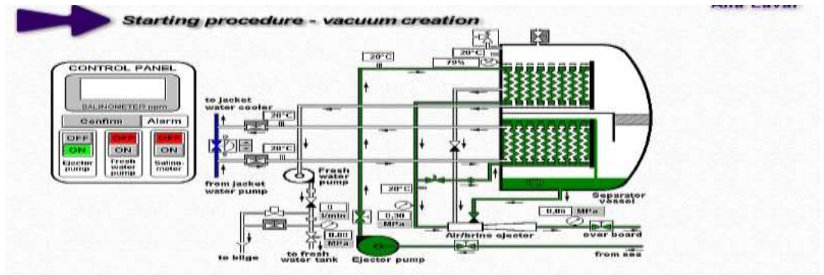
Gambar 2 Instalasi pada proses pembuat air tawar ( Fresh Water Generator )
